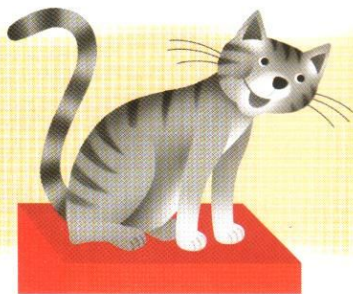
3. cat
