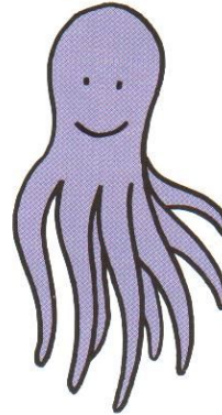
octopus
